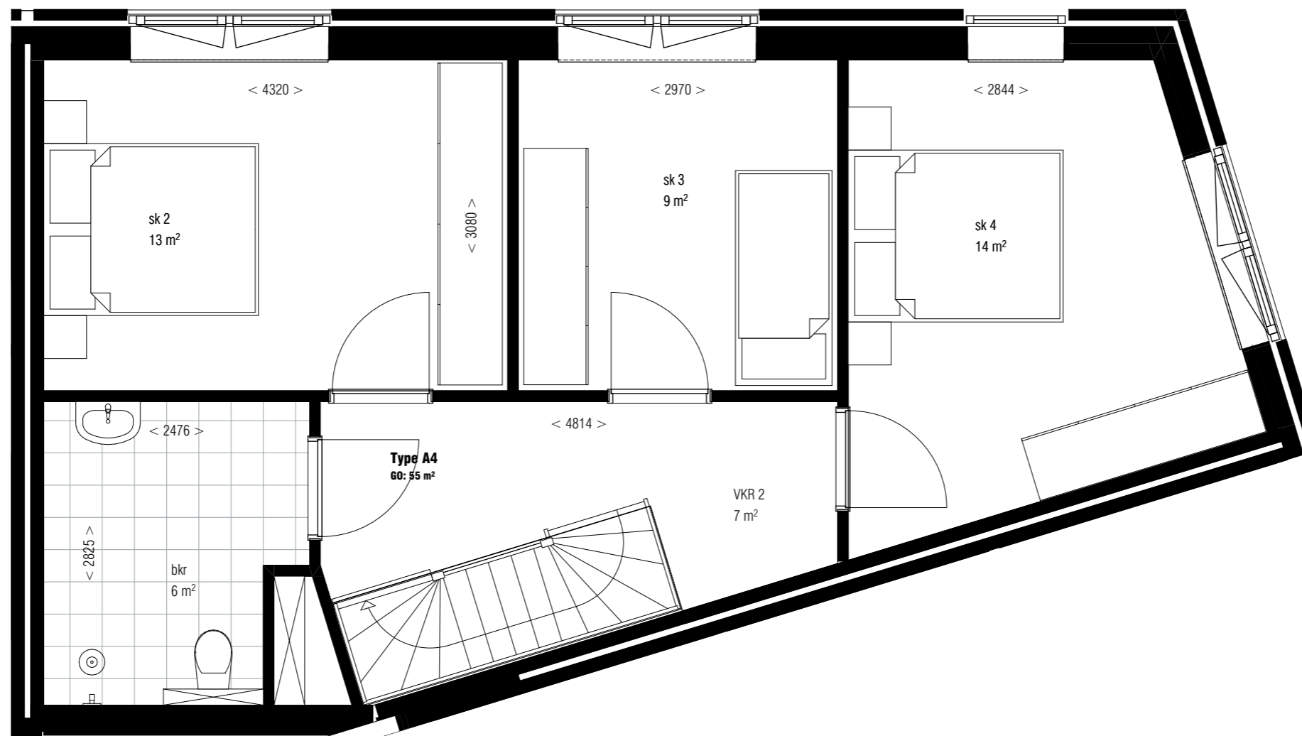
Type A4 2E VERDIEPING
